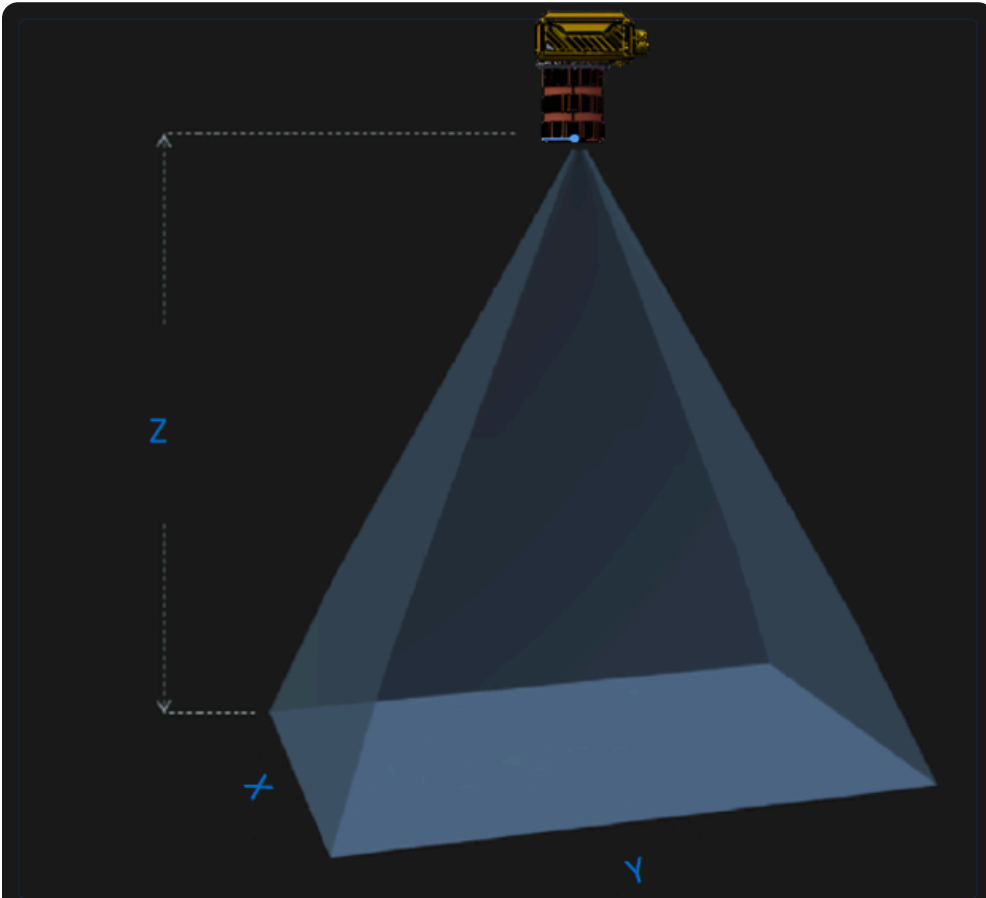
工作距离与视场关系示意图 A(工作距离) = 284mm, B(视野宽度) = 100mm, C(视野长度) = 100mm
