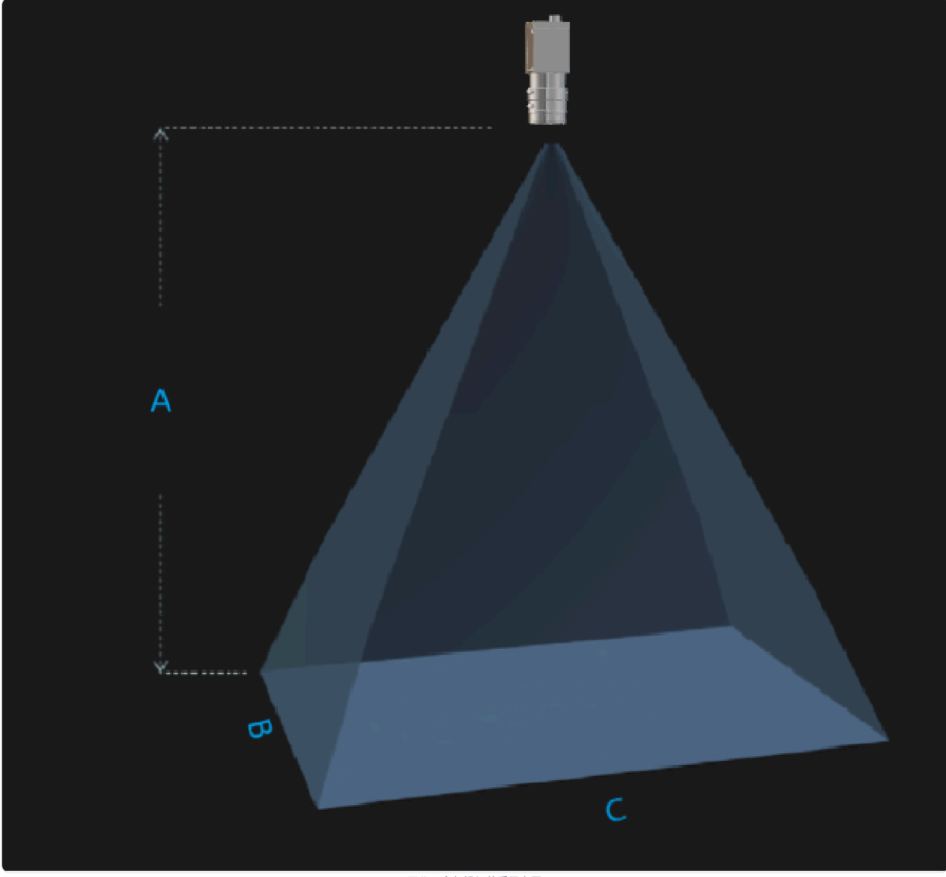
工作距离与视场关系示意图 A(工作距离) = 100mm, B(视场宽度) = 20mm, C(视场长度) = 20mm
