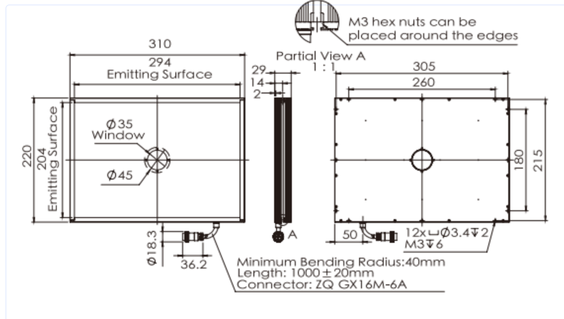
光源尺寸图
