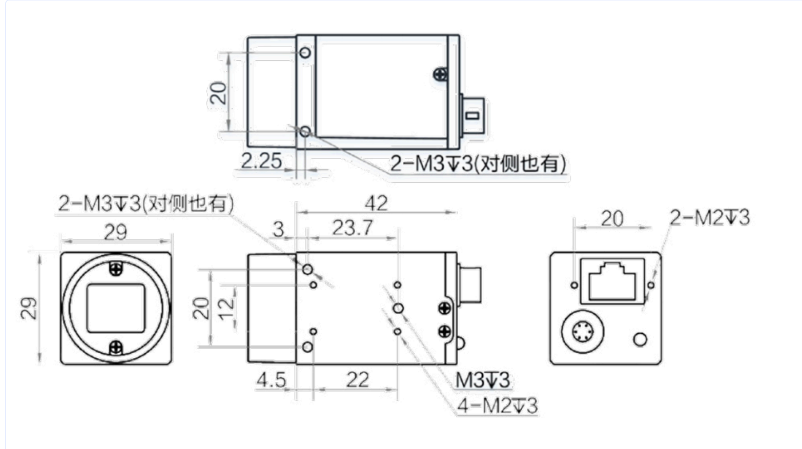
相机尺寸图
