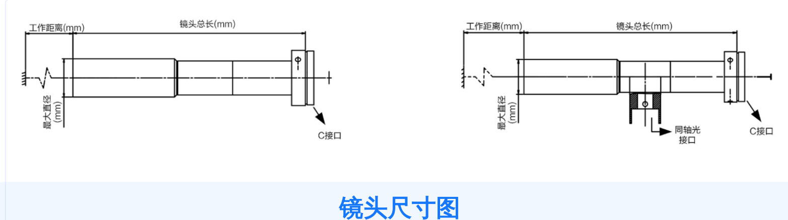
镜头尺寸图
