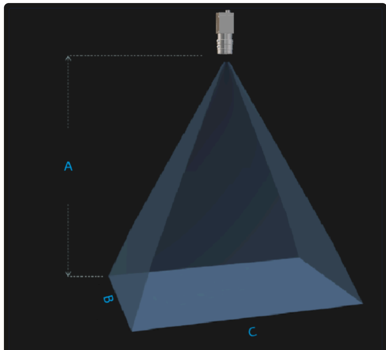
工作距离与视场关系示意图 A(工作距离) = 449mm, B(视野宽度) = 40mm, C(视野长度) = 200mm
