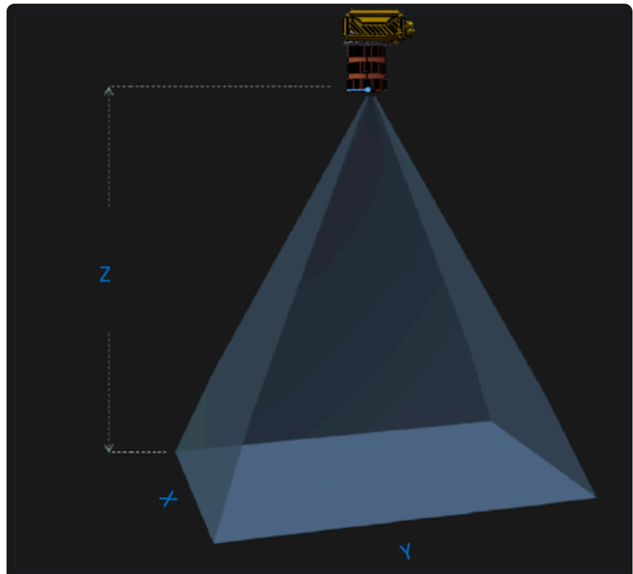
工作距离与视场关系示意图 A(工作距离) = 438mm, B(视野宽度) = 75mm, C(视野长度) = 220mm
