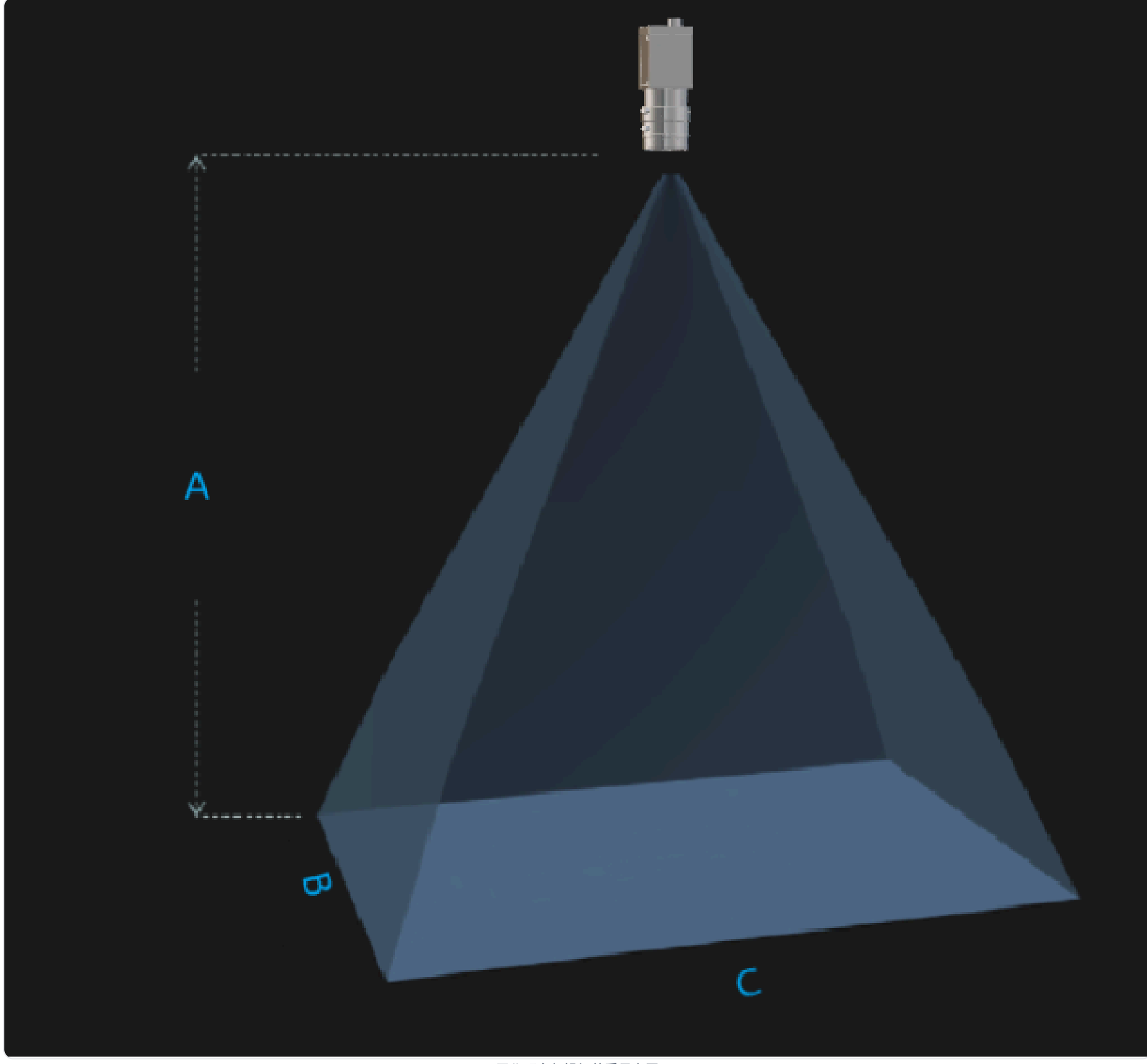
工作距离与视场关系示意图 A(工作距离) = 294mm, B(视野宽度) = 100mm, C(视野长度) = 100mm
