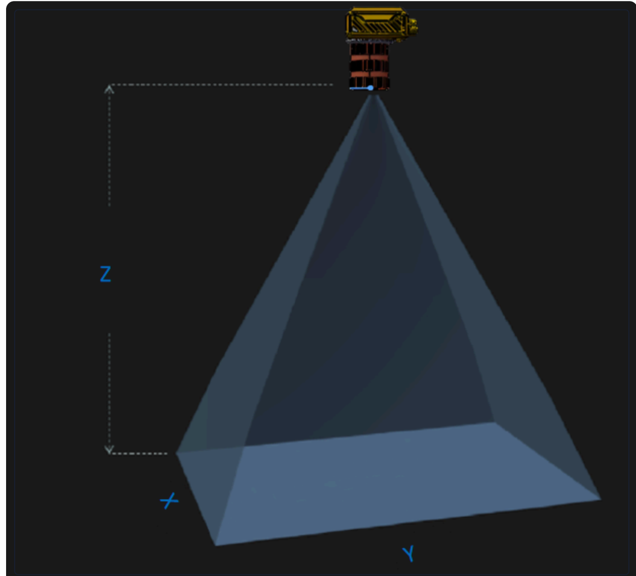
工作距离与视场关系示意图 A(工作距离) = 109mm, B(视野宽度) = 12mm, C(视野长度) = 15mm
