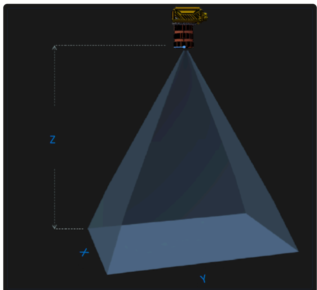
工作距离与视场关系示意图 A(工作距离) = 175mm, B(视野宽度) = 60mm, C(视野长度) = 60mm
