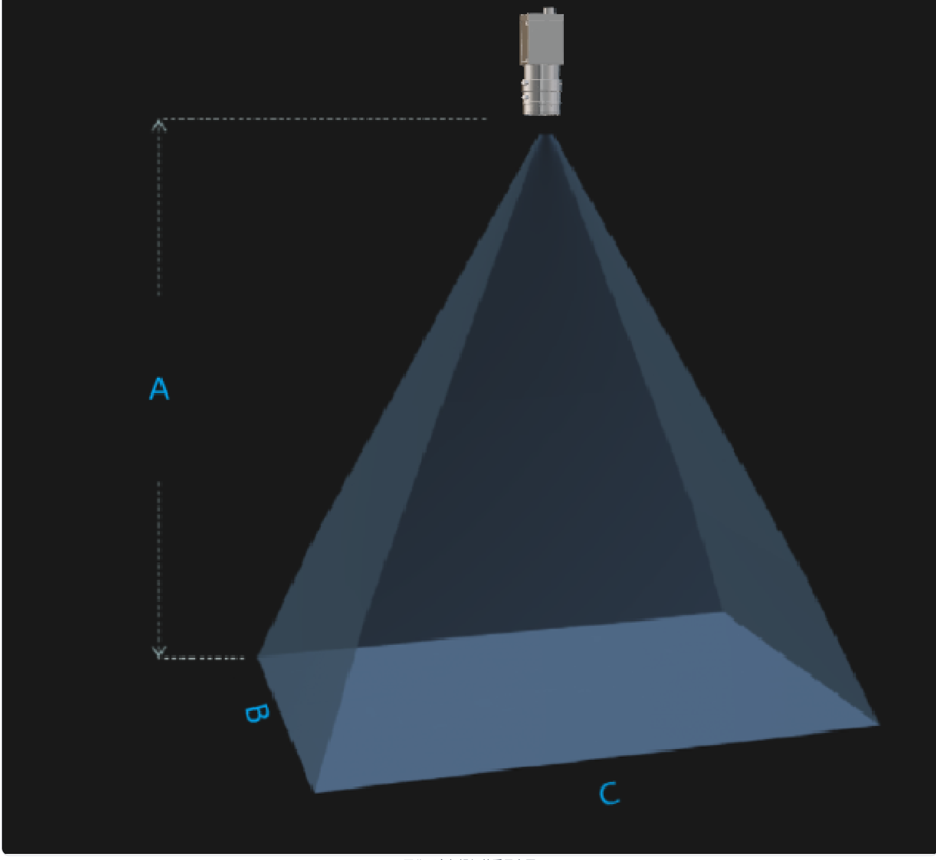
工作距离与视场关系示意图 A(工作距离) = 131mm, B(视场宽度) = 20mm, C(视场长度) = 20mm
