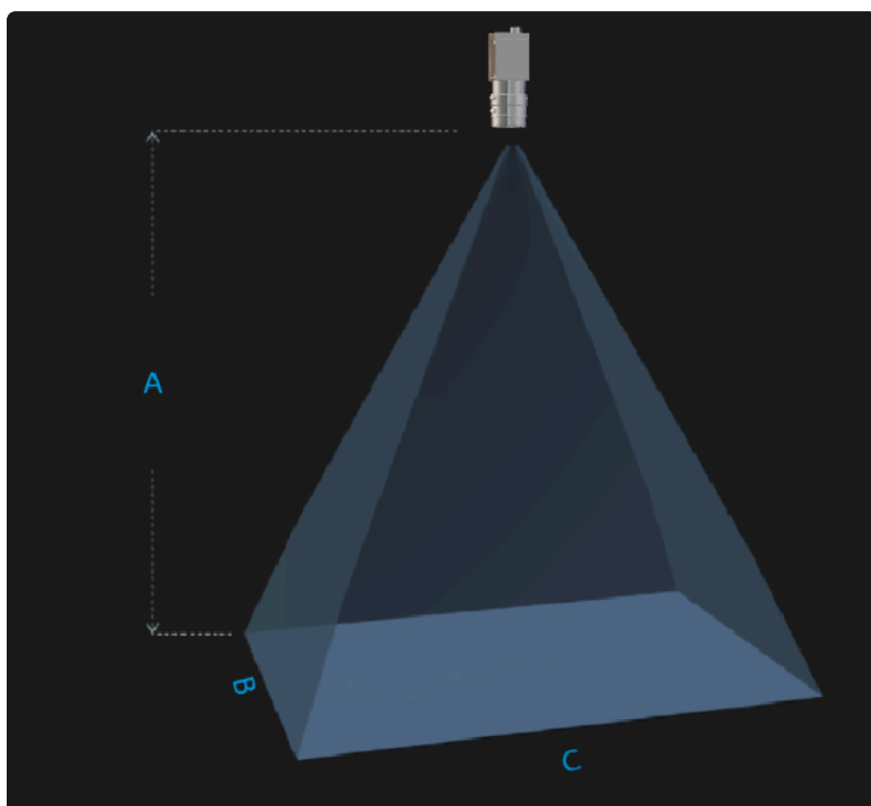
图2：相机工作距离与视场关系 A(高) = 600mm, B(宽) = 200mm, C(长) = 300mm
