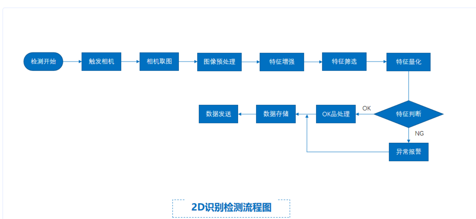
2D识别检测流程图
