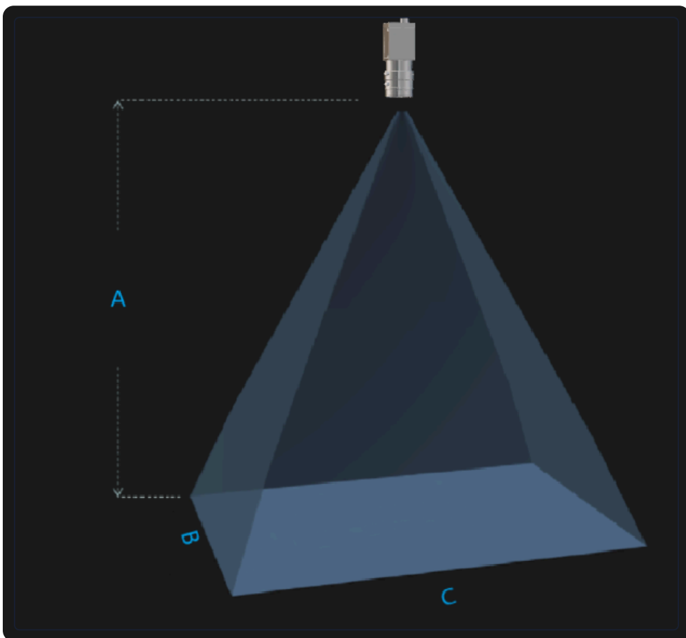
工作距离与视场关系示意图 A(工作距离) = 1209mm, b(视野宽度) = 960mm, c(视野长度) = 1600mm
