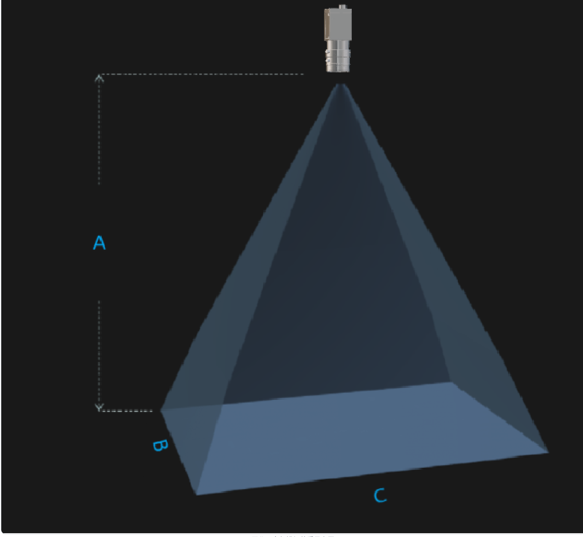
工作距离与视场关系示意图 A(工作距离) = 184mm, B(视场宽度) = 50mm, C(视场长度) = 50mm
