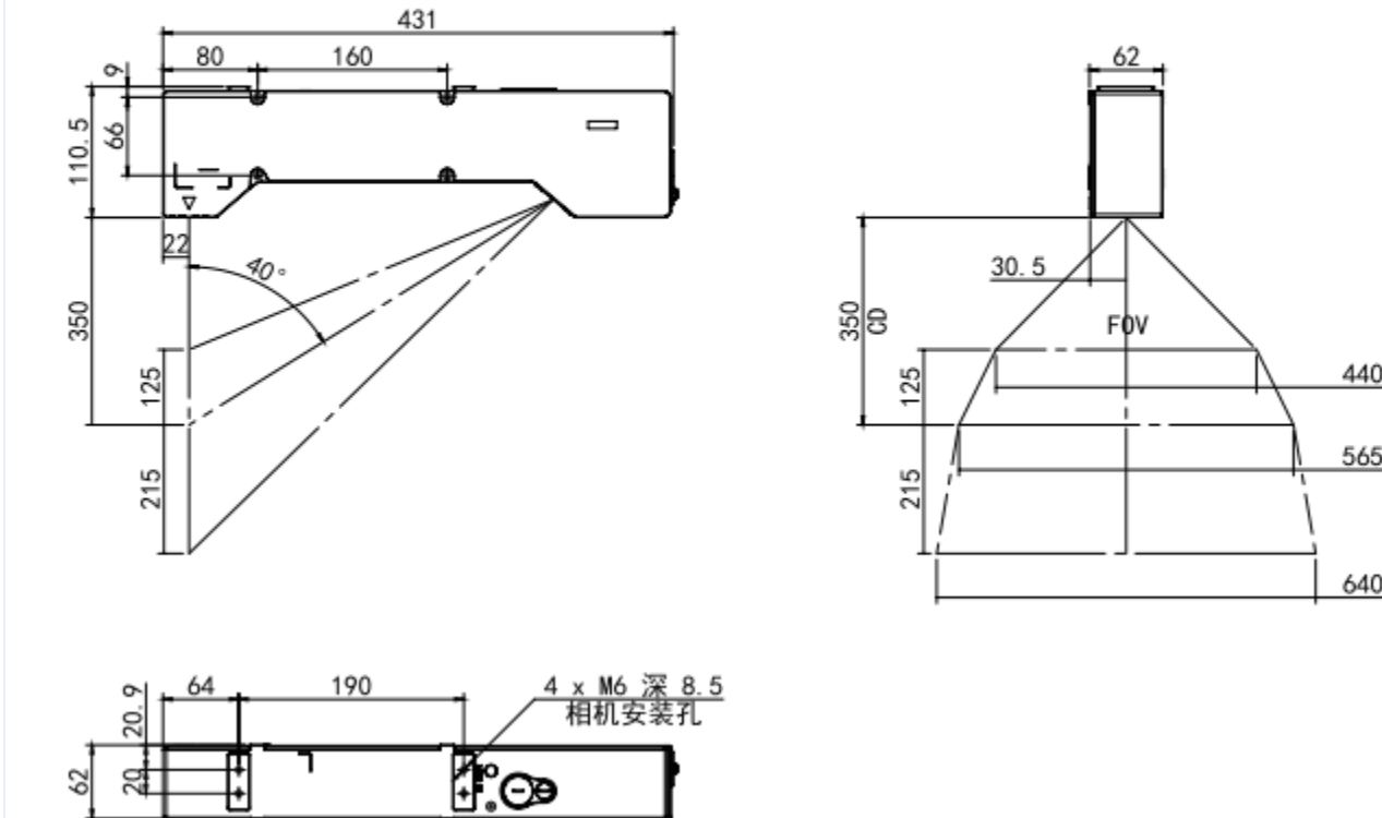
镜头尺寸图
