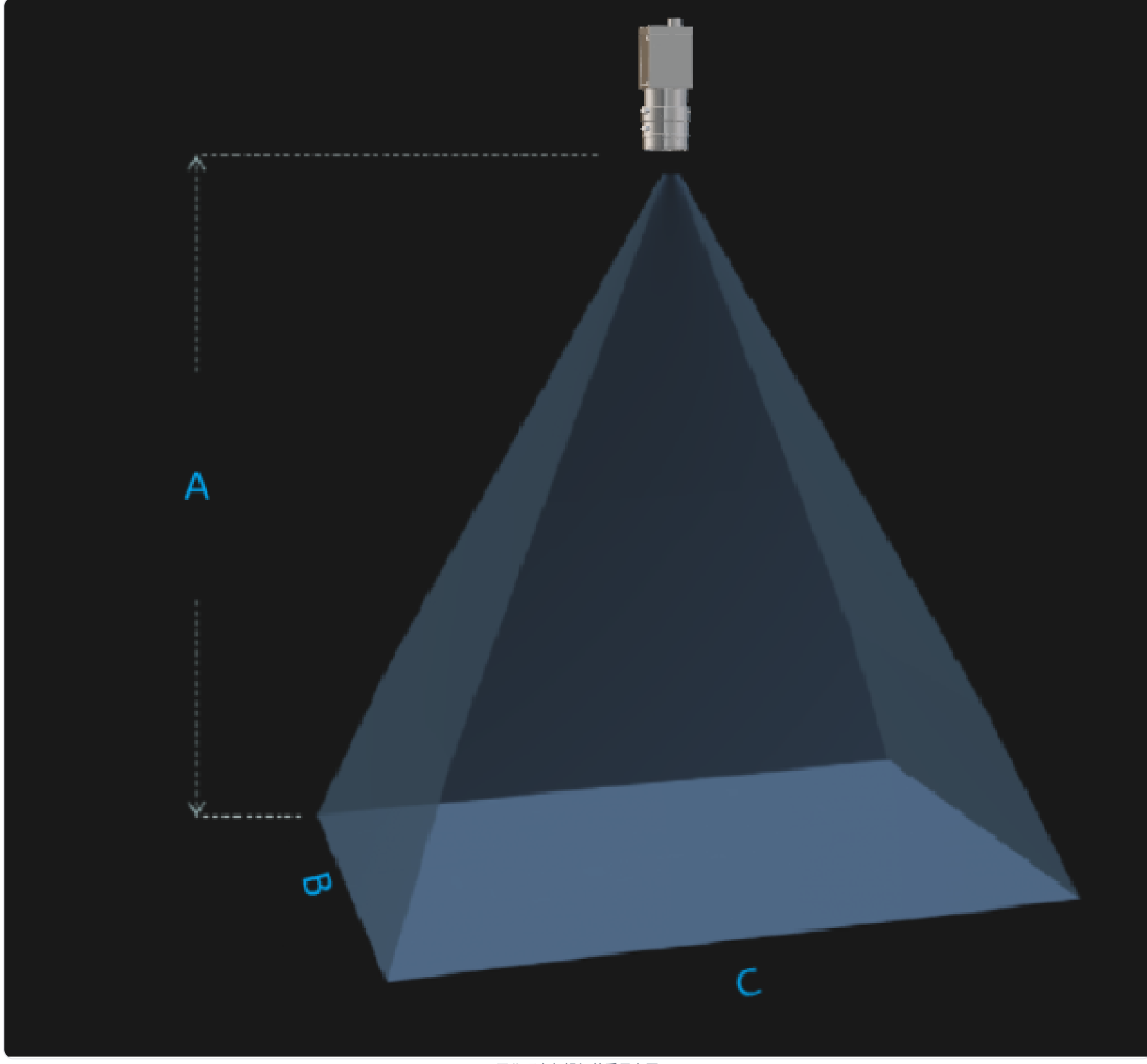
工作距离与视场关系示意图 A(工作距离) = 131mm, B(视场宽度) = 20mm, C(视场长度) = 20mm
