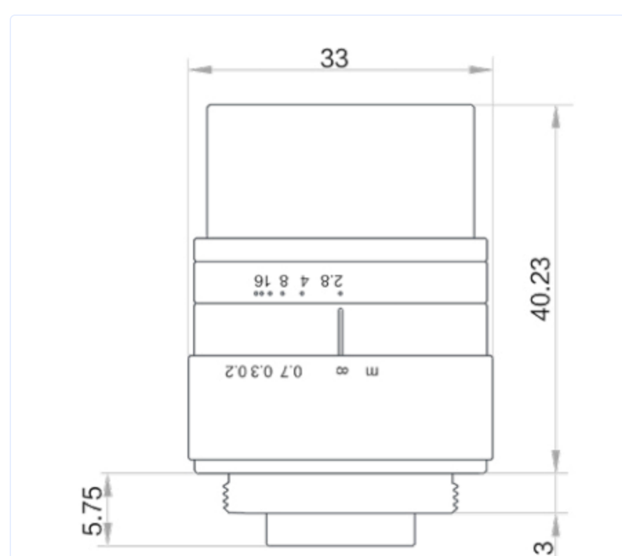
镜头尺寸图
