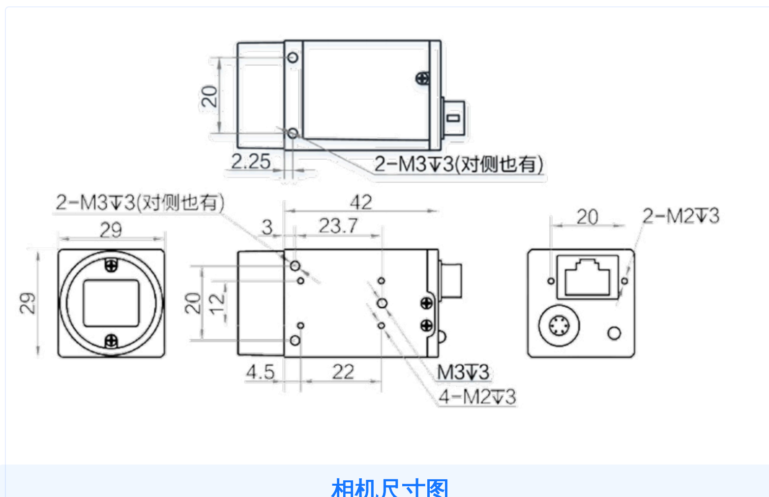
相机尺寸图
