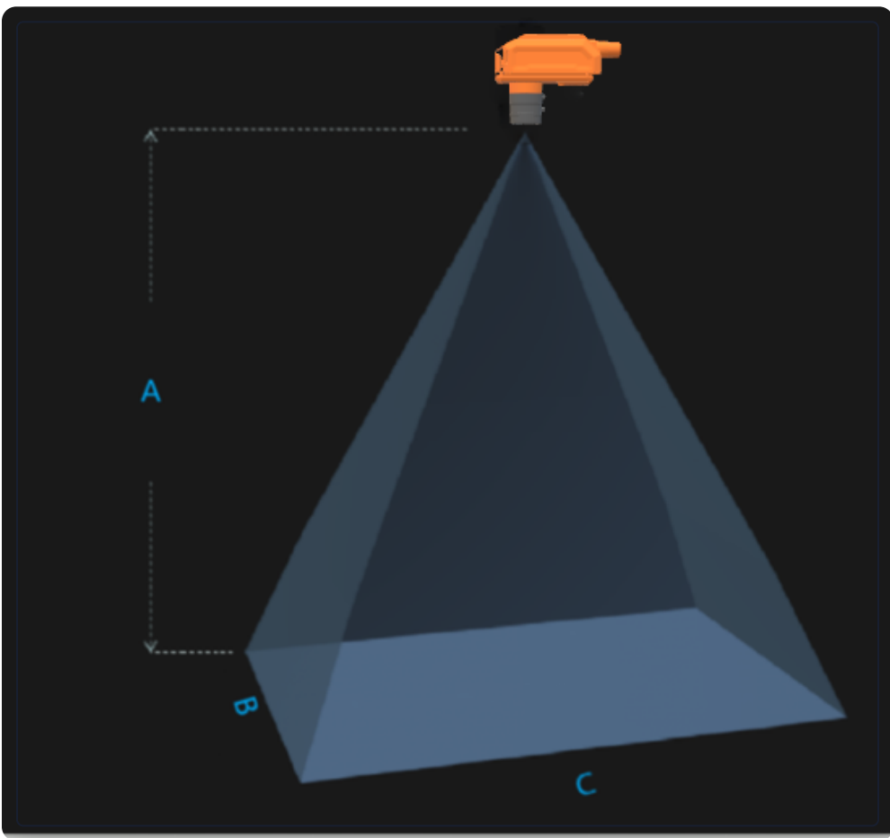
工作距离与视场关系示意图 A(工作距离) = 555mm, X(视野宽度) = 150mm, Y(视野长度) = 200mm
