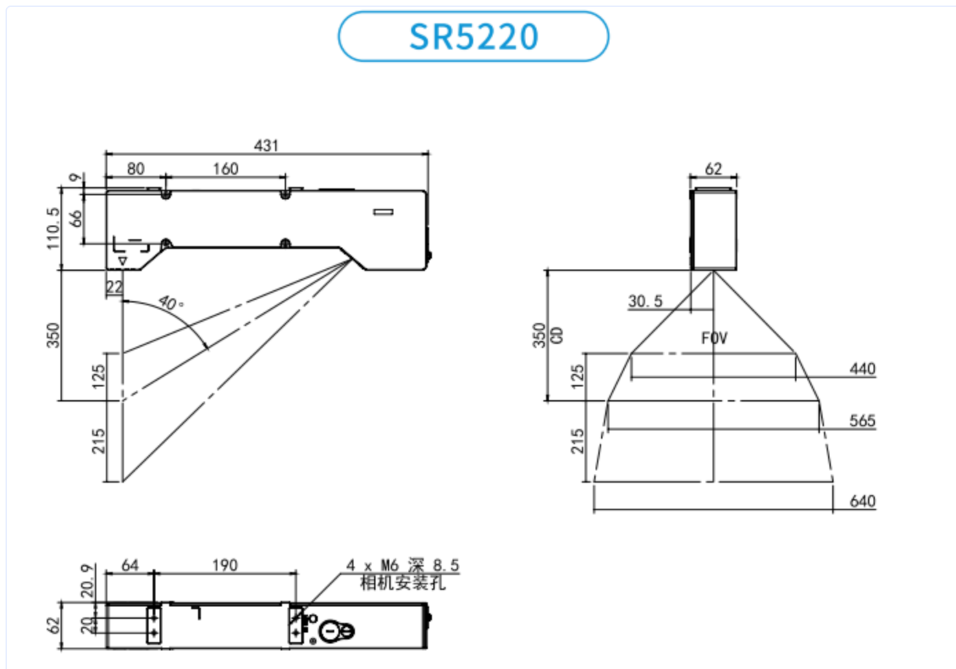
镜头尺寸图
